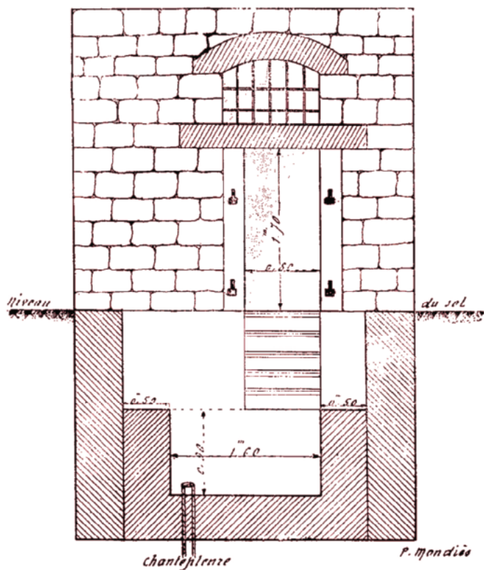
L'ENTRÉE DE LA SOURCE ET LE BASSIN DE CAPTATION EN SOUS-SOL
