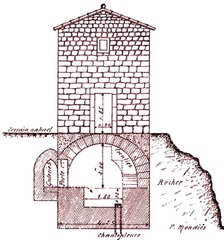
ÉLEVATION DE LA CABANE ET COUPE DU BASSIN DE RECUEILLEMENT EN SOUS-SOL
